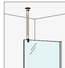
Suporte ao teto
